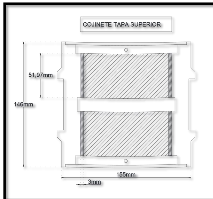
Fig.2 Plano longitudinal de tapa superior del Cojinete.
