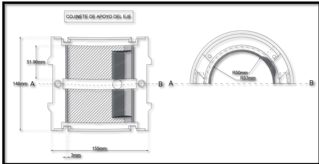
Fig.1 Plano longitudinal y transversal de tapa de apoyo del Cojinete.
