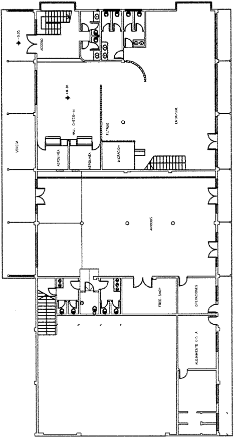
AEROESTACION PLANTA BAJA
