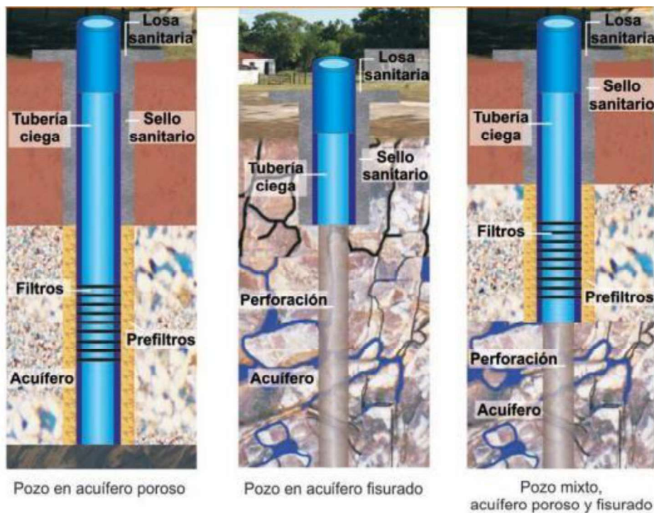
Figura Nr.2 Diseño del pozo.
