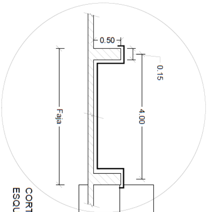
CORTE TRANSVERSAL ESQUEMÁTICO esc. 1/150
