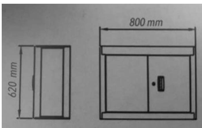
Imagen 1- Modular aéreo modo ejemplo.
