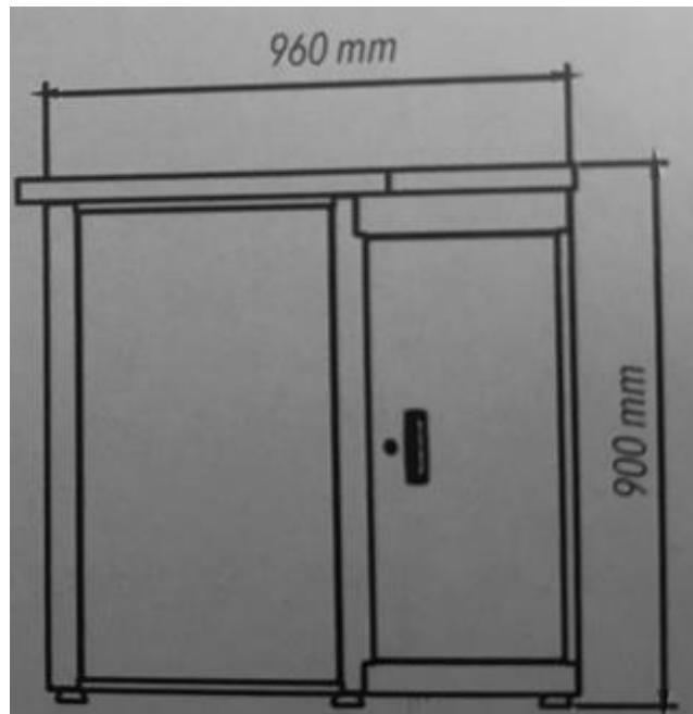
Imagen 4- Mesa de trabajo en L con armario ejemplo.
