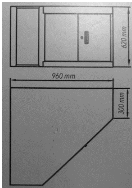
Imagen 2- Modular aéreo en L modo ejemplo.
