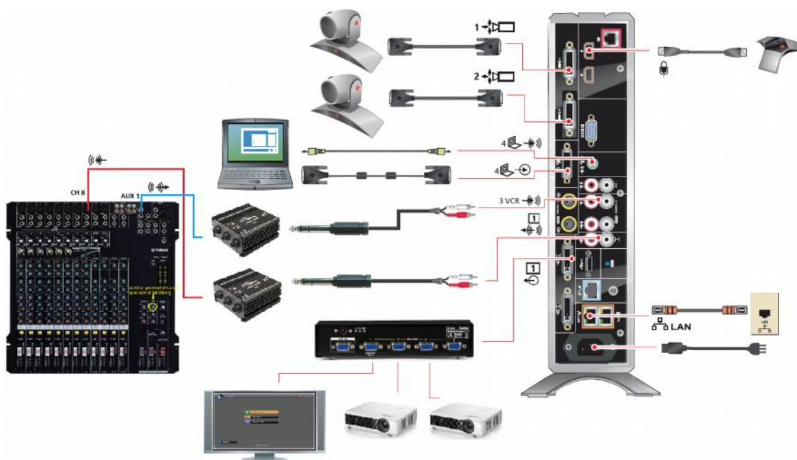
Figura 1: Conexionado de parte del equipamiento existente, a modo ilustrativo
