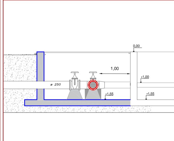
D 1 - CORTE A-A
