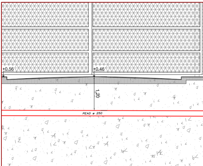
D 2 - CORTE B-B
