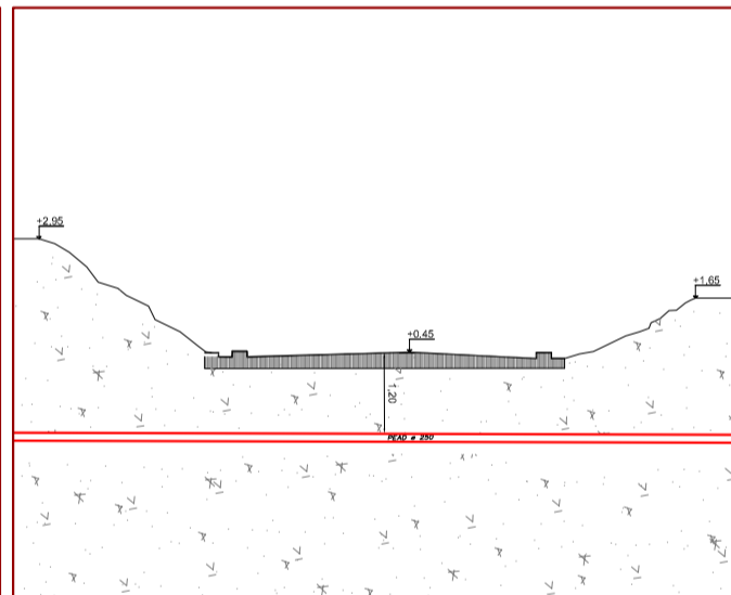
D 3 - CORTE C-C
