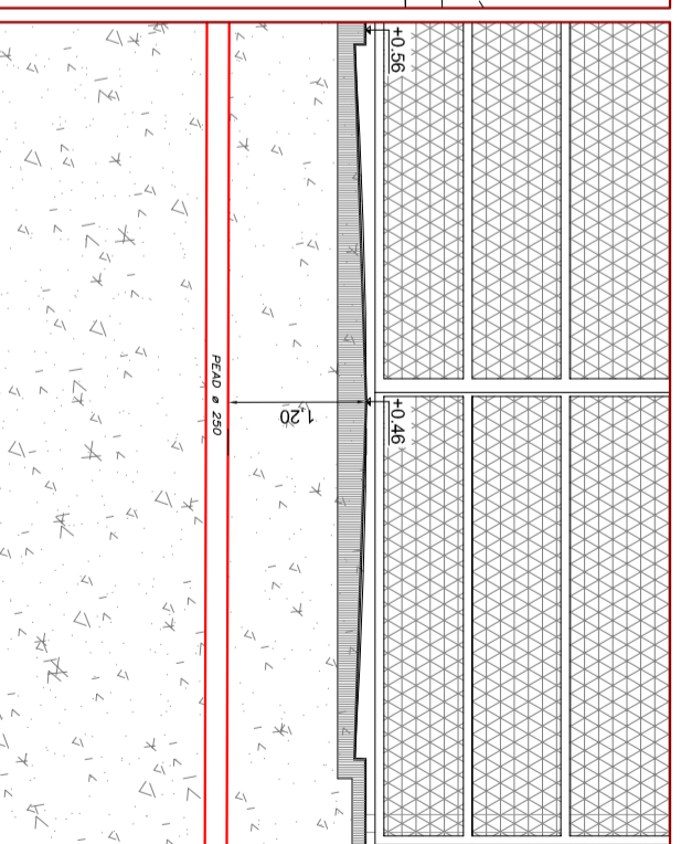
D 2 - CORTE B-B
