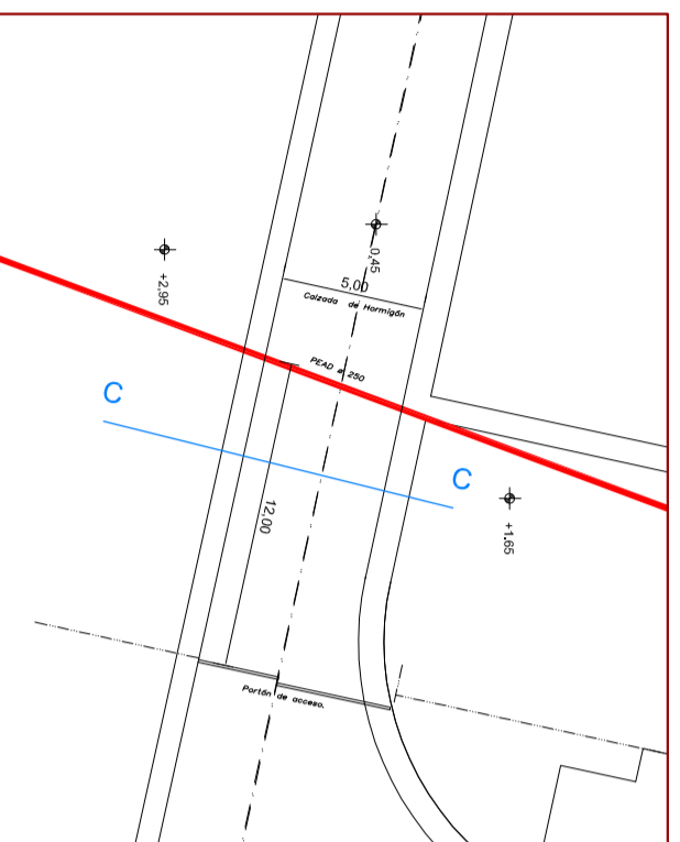
D 3 - PLANTA
