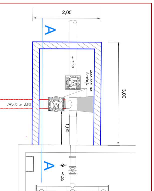
D 1 - PLANTA
