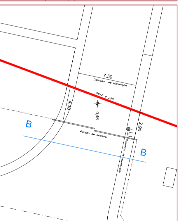
D 2 - PLANTA
