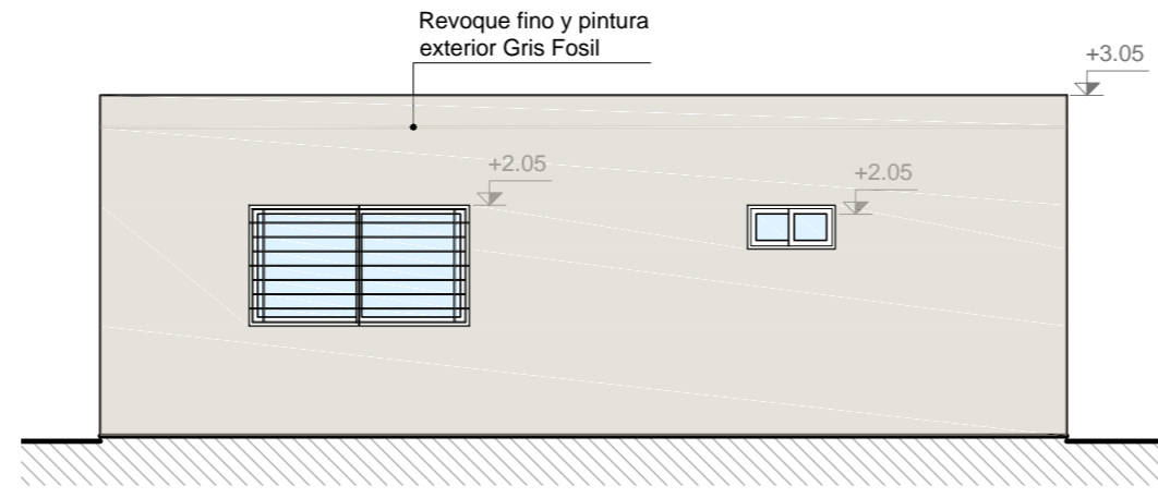
FACHADA POSTERIOR
