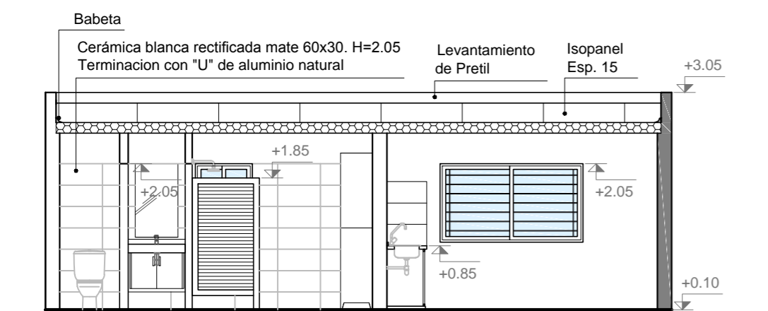
CORTE A-A
