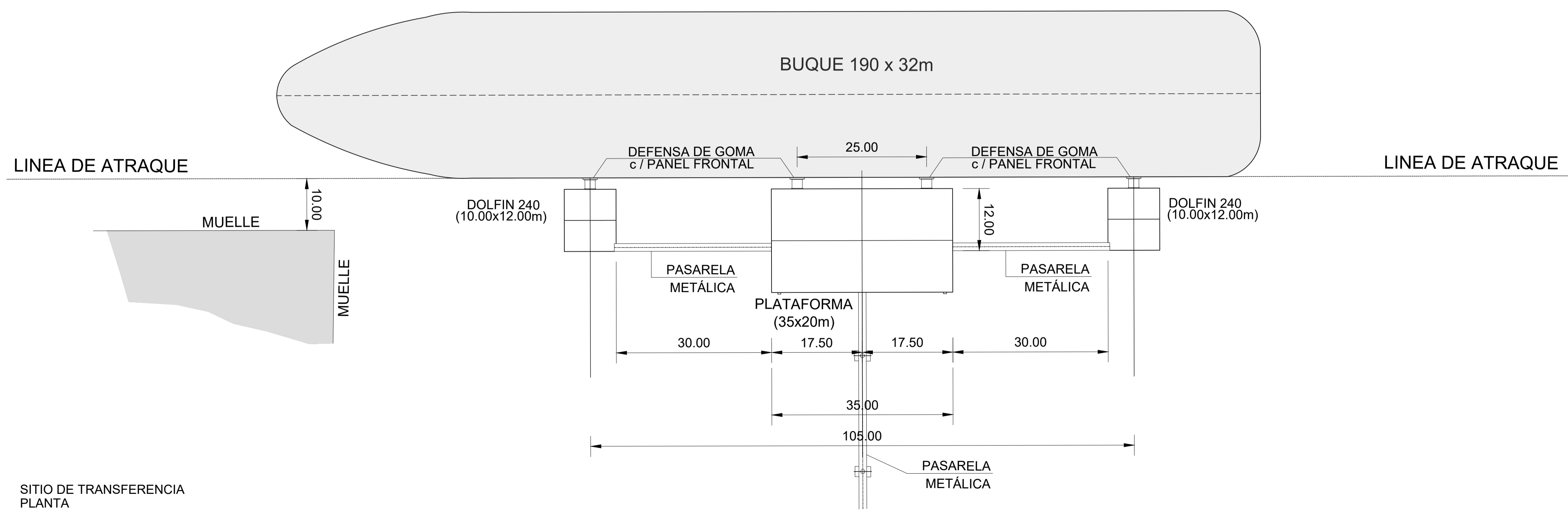
SITIO DE TRANSFERENCIA LAYOUT GENERAL ESCALA 1:1250
