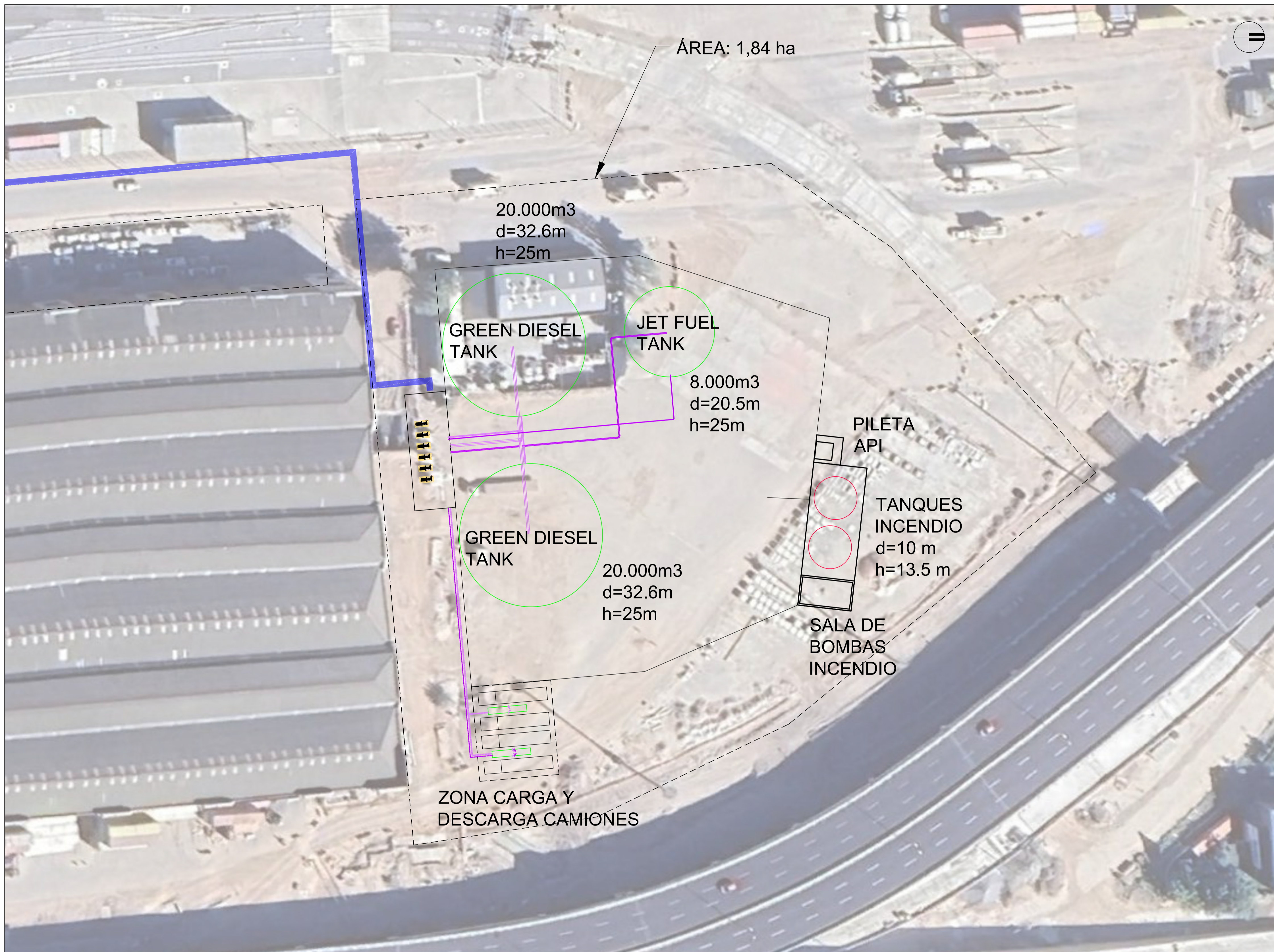
ZONA DE ALMACENAMIENTO LAYOUT GENERAL ESCALA 1:500
