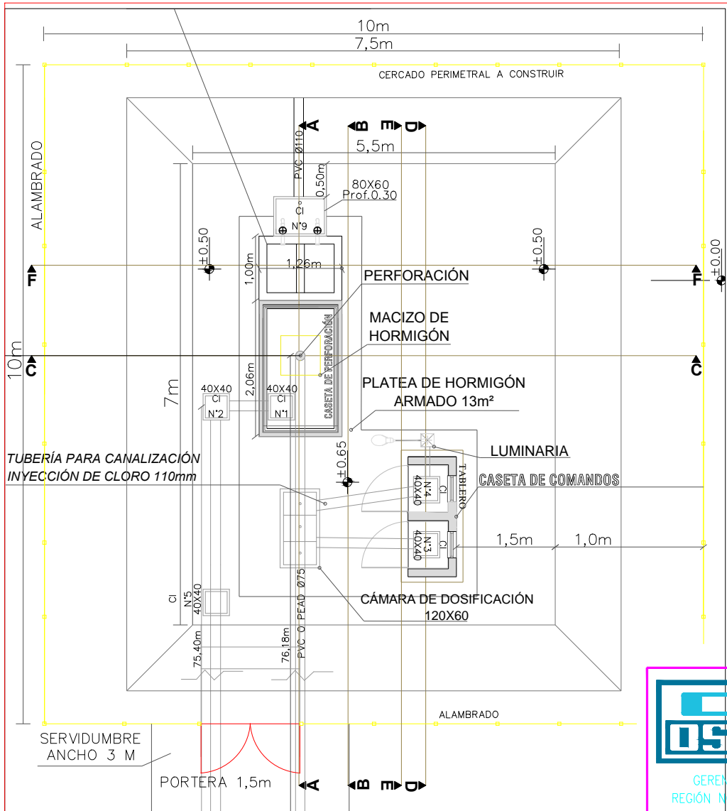
PLANTA DETALLE ESCALA 1:50
