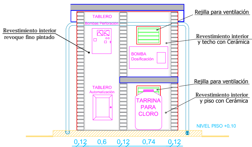
CORTE D-D
