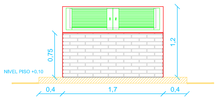
CORTE B-B
