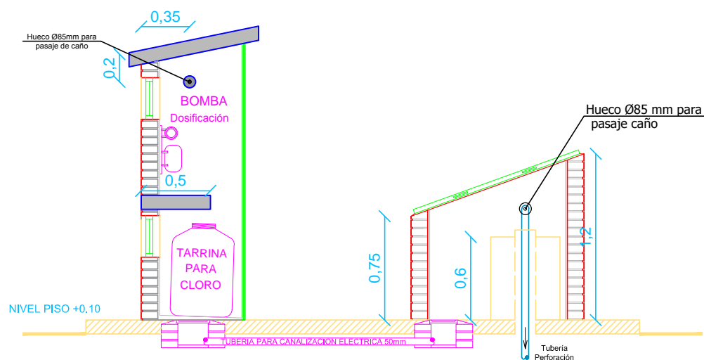
CORTE C-C
