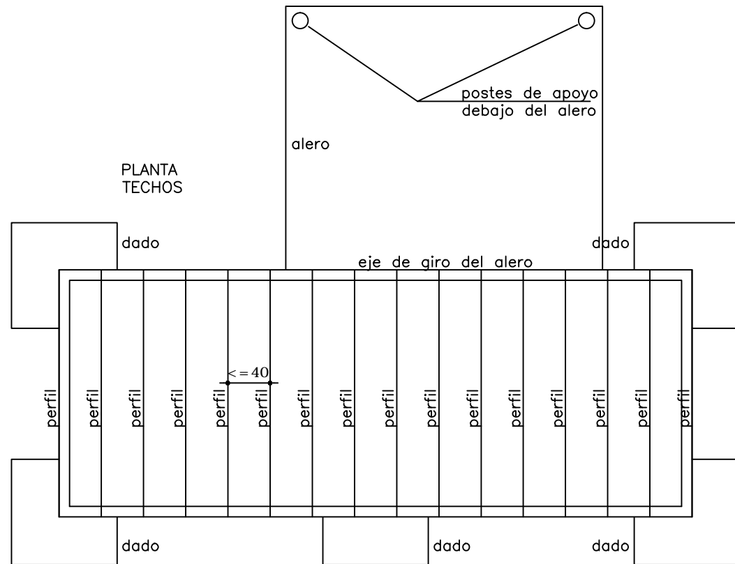
PLANTA TECHOS 1/50
