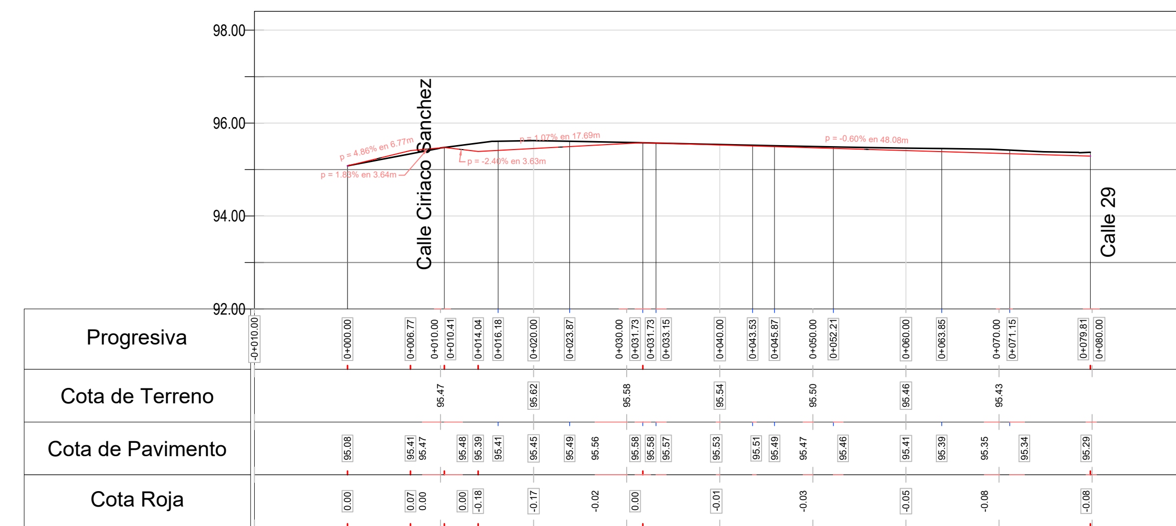
Perfil Longitudinal: Calle Union_1; deformacion H:V = 5
