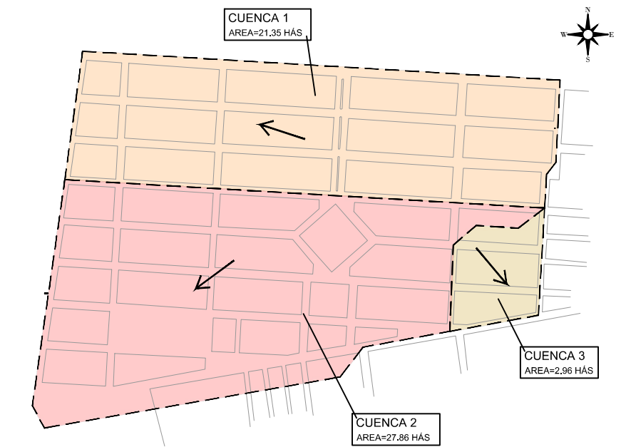
MACROCUCENAS DE DRENAJE ESC: 1:10000
