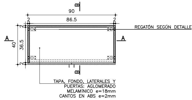
PLANTA esc 1:20
