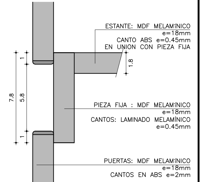
DETALLE 1 esc 1:2
