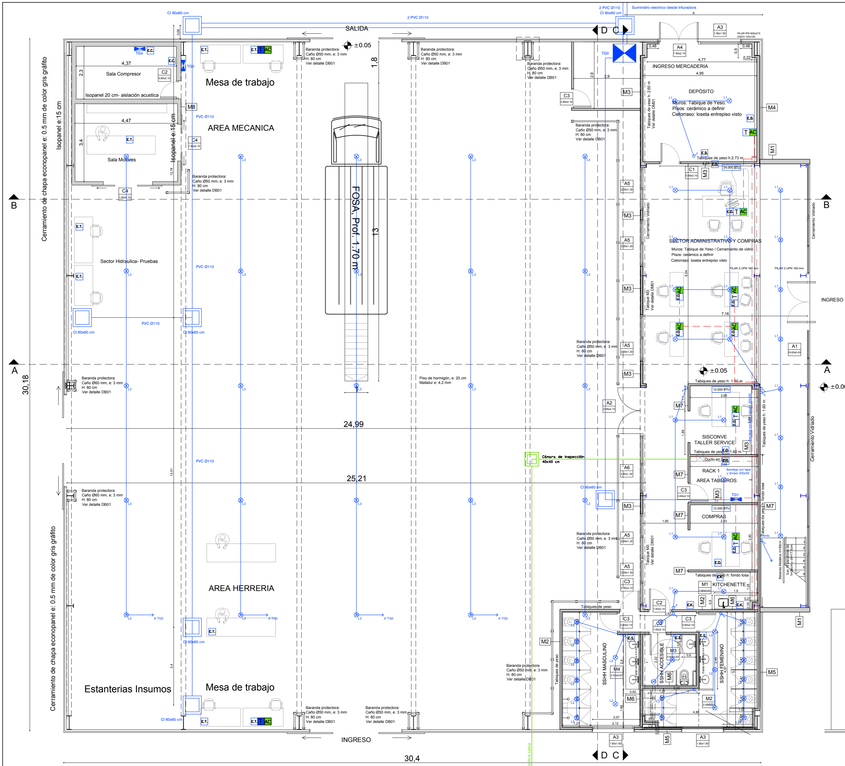
PLANTA BAJA DE ALBAÑILERIA
