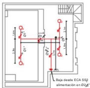
Subsuelo 4
