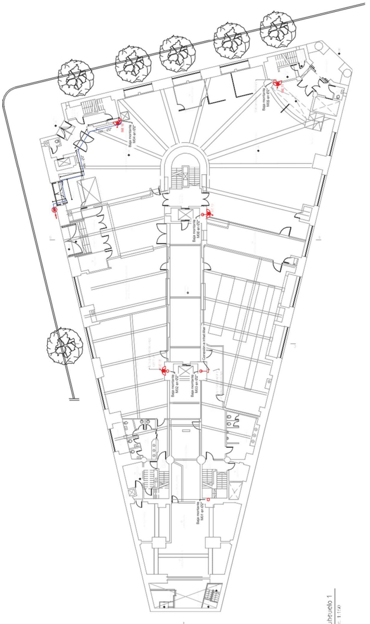
Subsuelo 2 Esc. 1:150
