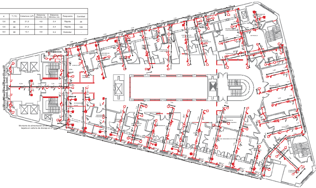
Piso 7 Escala: 1:150
