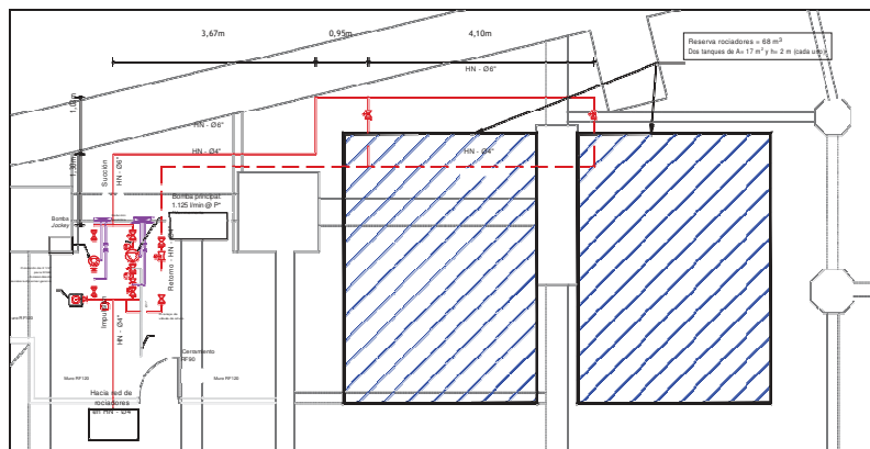
Esquema sala de bombas y reserva Esc. 1:50
