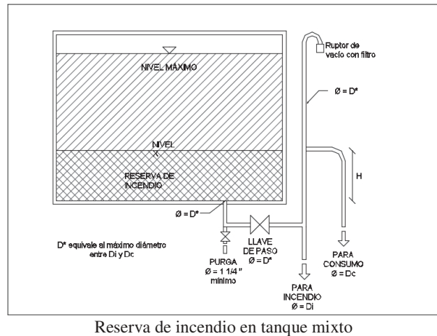
Reserva de incendio en tanque mixto
