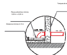
Esquema de toma - placa antivórtice Esc. 1:50
