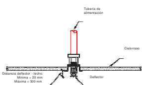
Esquema ilustrativo - Rociador colgante
