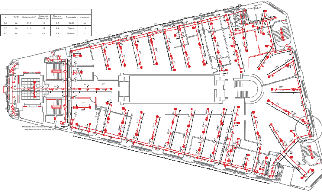
Piso 5 Esc. 1:150
