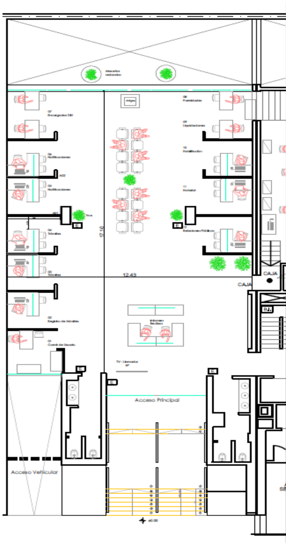
PLANTA DE ALBAÑILERÍA HALL PRINCIPAL
