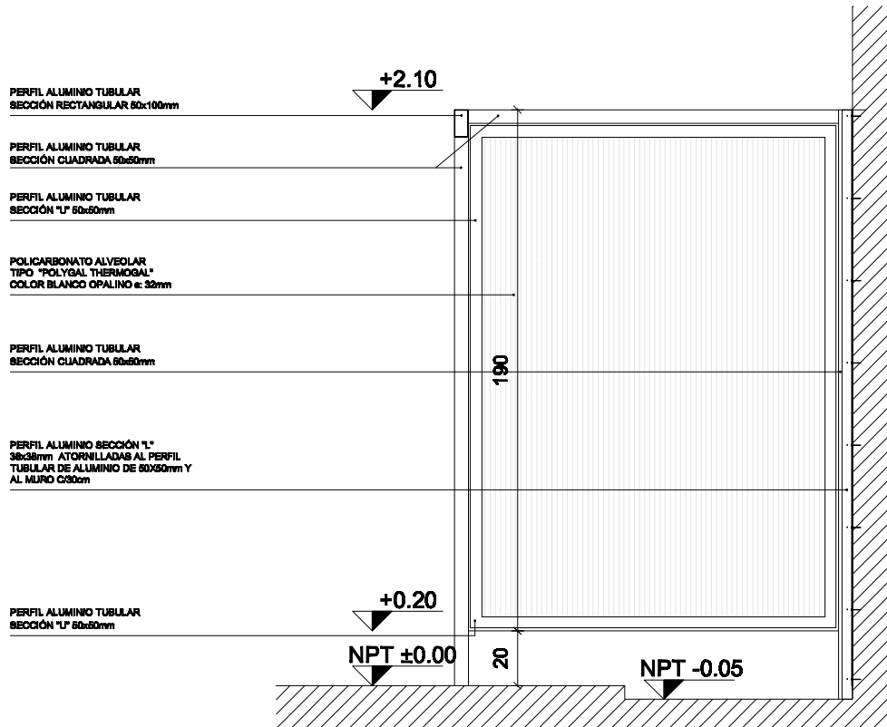
CORTE 1-1 | 2-2
