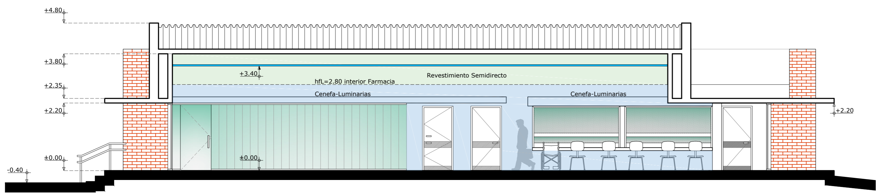
CORTE A-A FARMACIA
