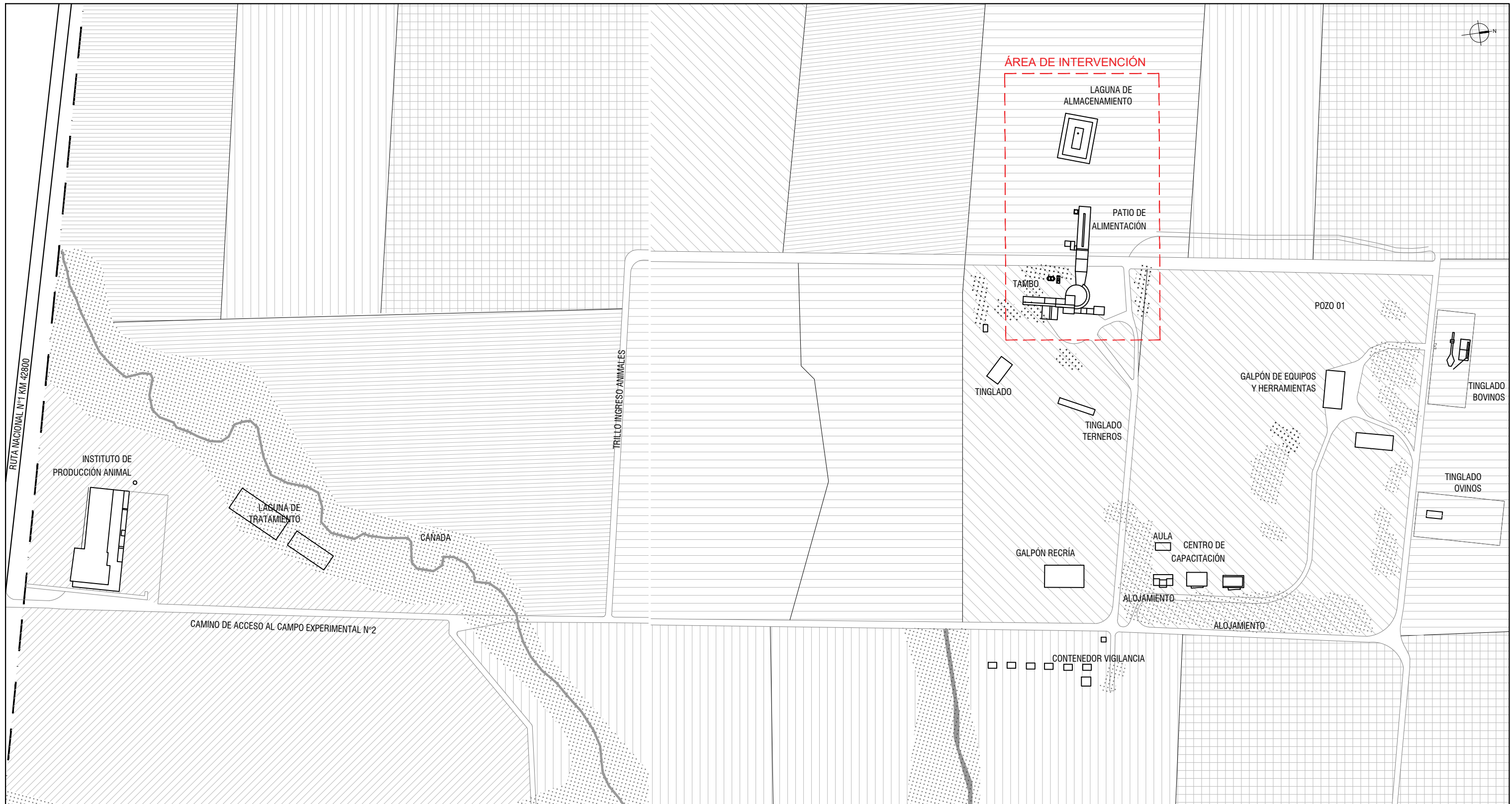
PLANTA DE UBICACIÓN / ÁREA DE INTERVENCIÓN Esc 1:3000
