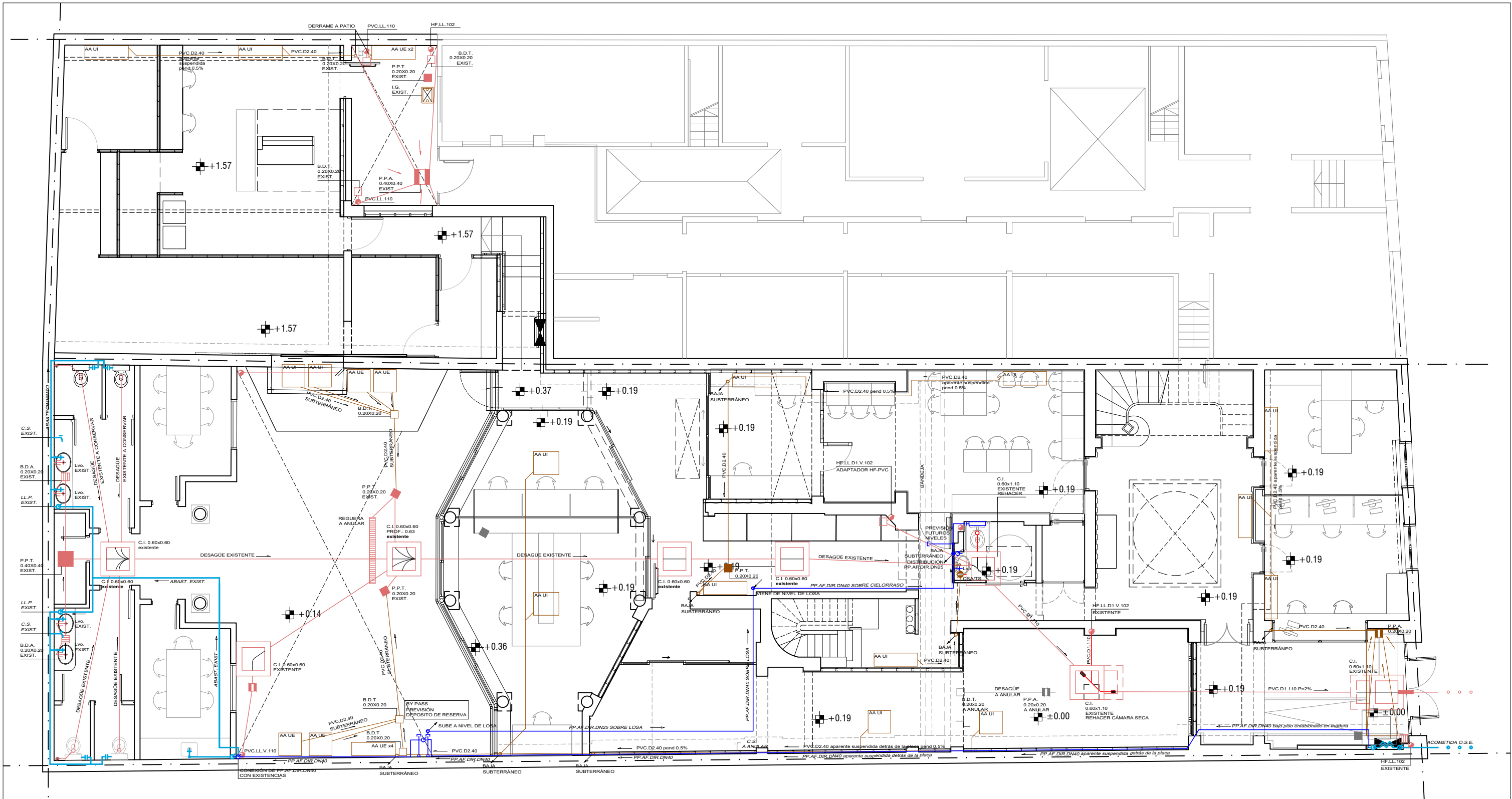
PLANTA BAJA Esc 1.100
