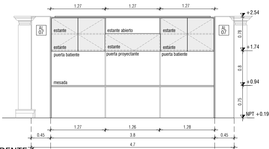
FRETE 1 Esc 1.50
