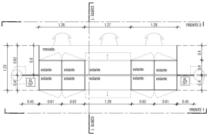
PLANTA Esc 1.50
