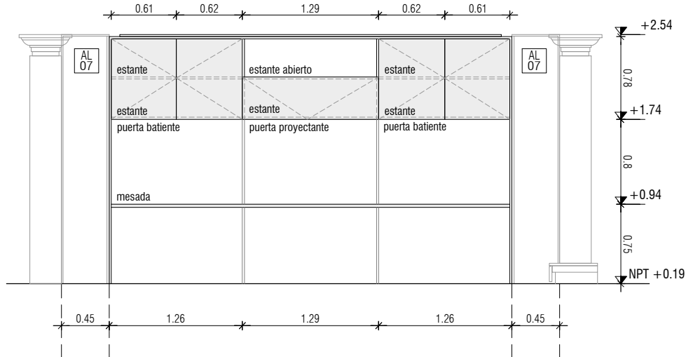
FRETE 2 Esc 1.50
