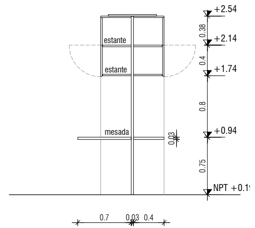
CORTE 1 Esc 1.50
