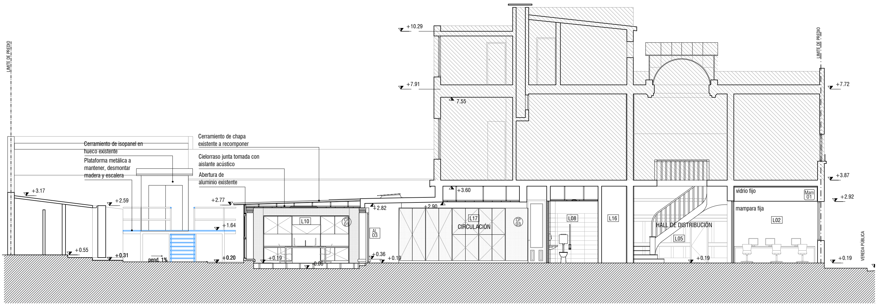
CORTE FF Esc 1:100
