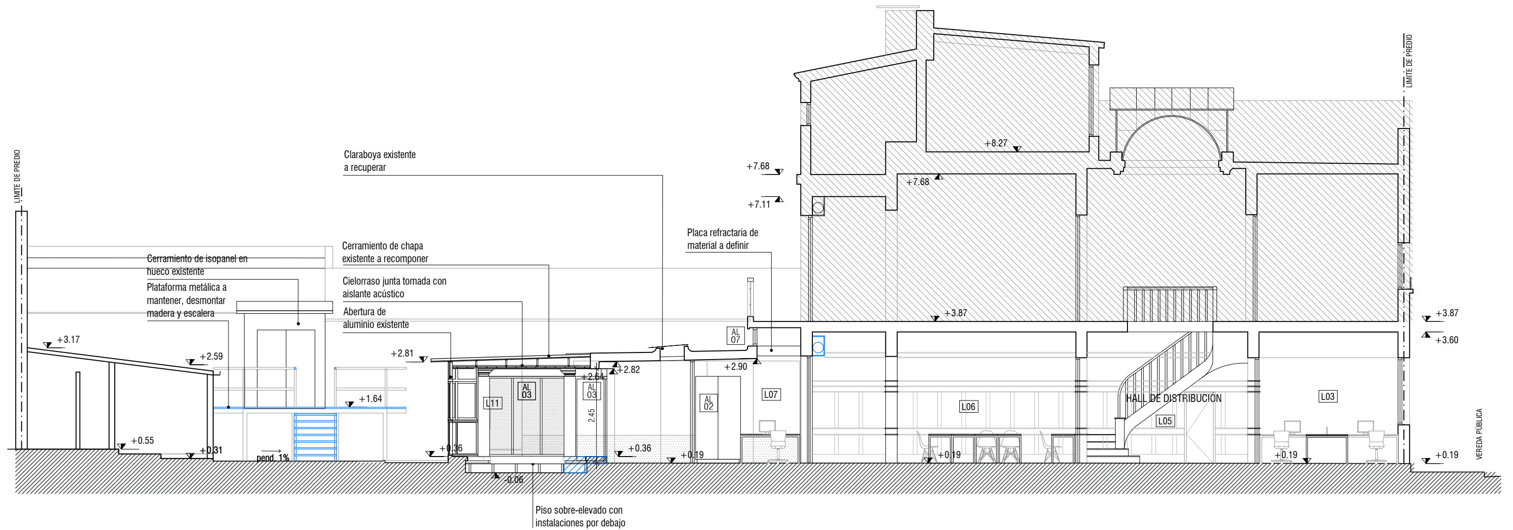
CORTE EE Esc 1:100
