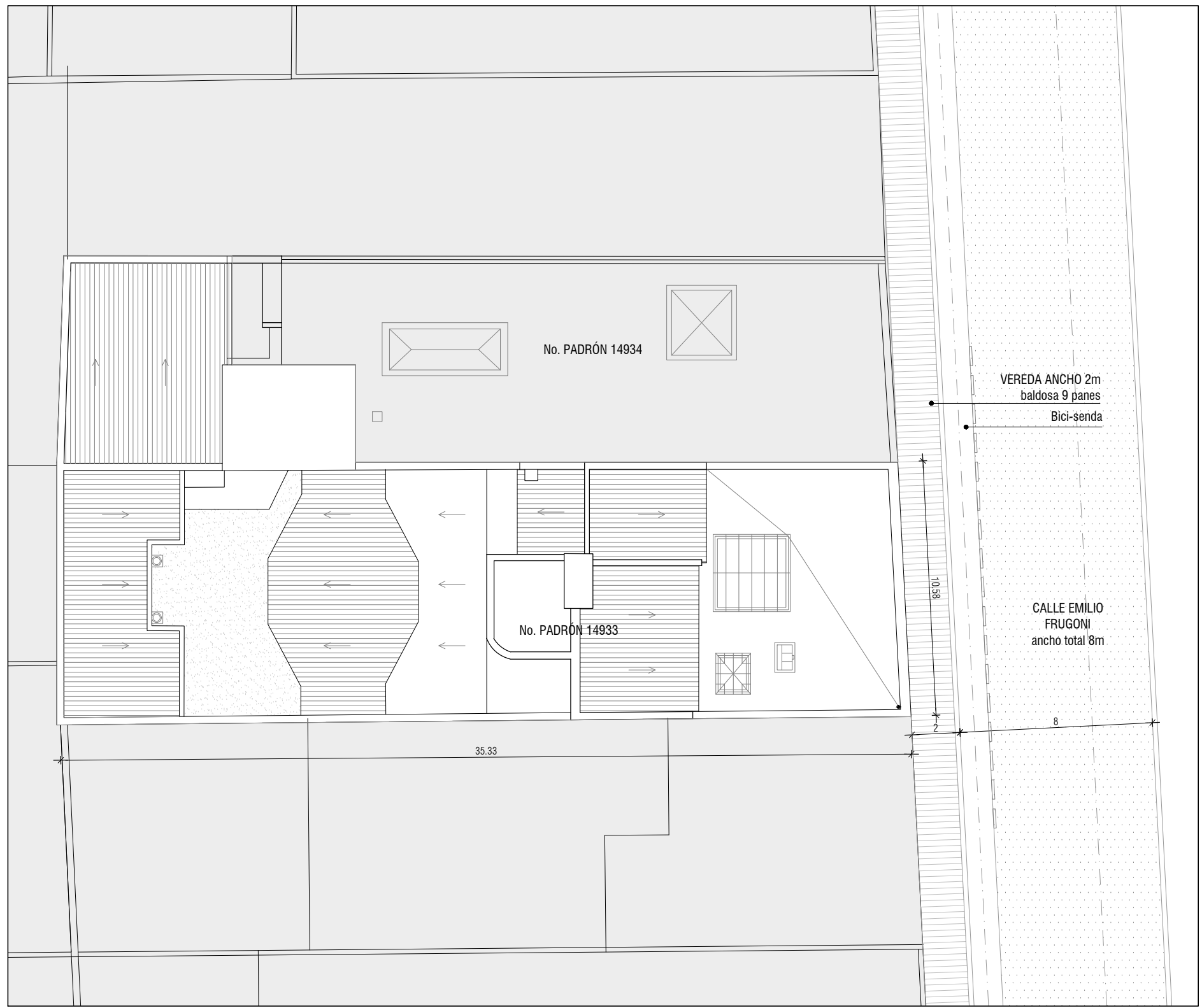
PLANTA IMPLANTACION Esc 1.200
