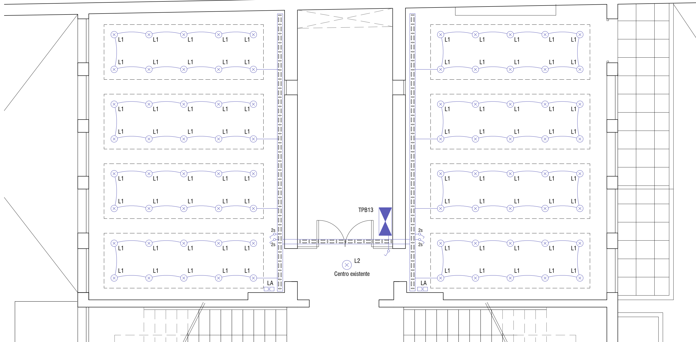
PLANTA ILUMINACIÓN esc. 1.50
