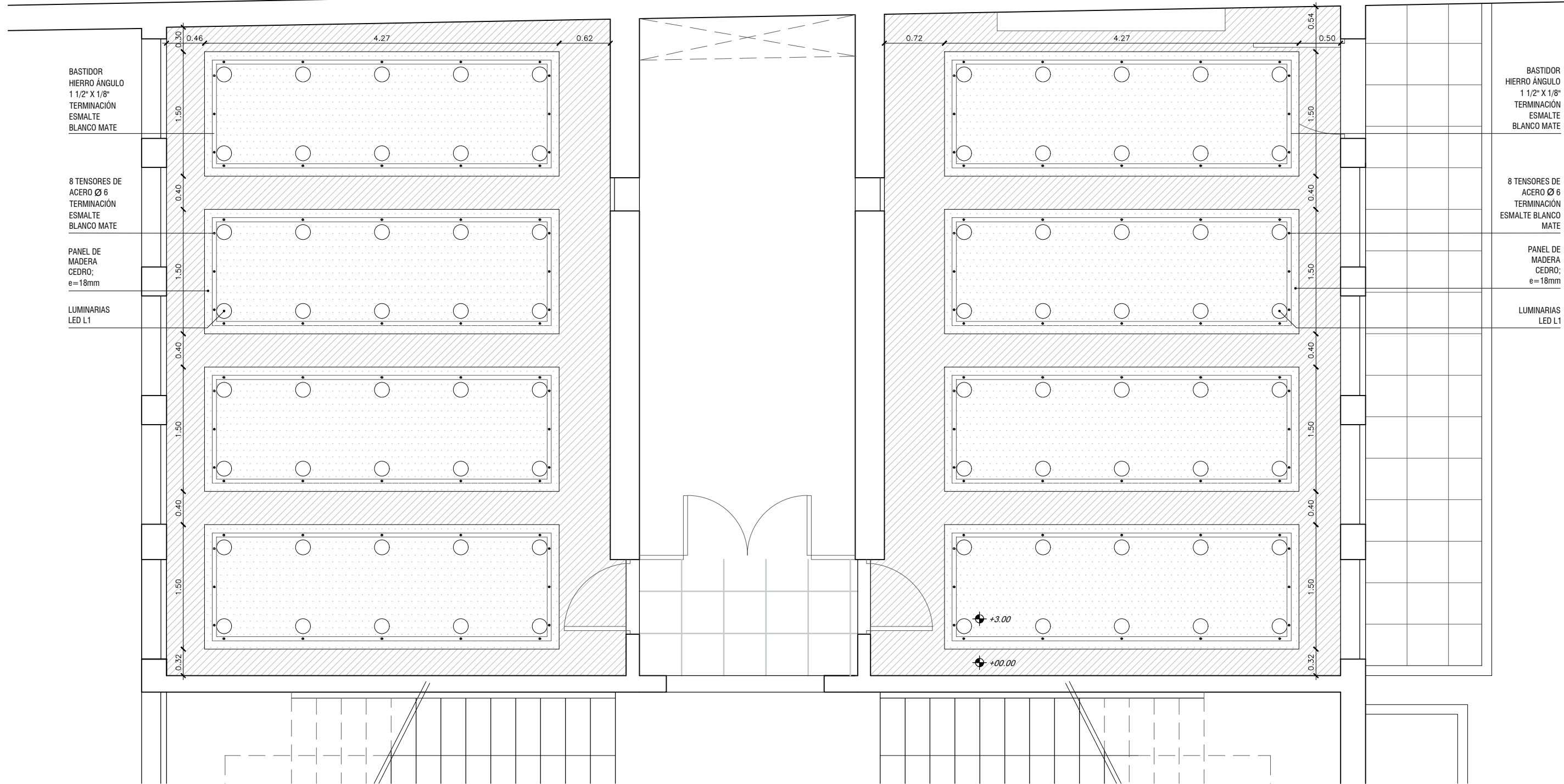
PLANTA CIELORRASO esc. 1.50
