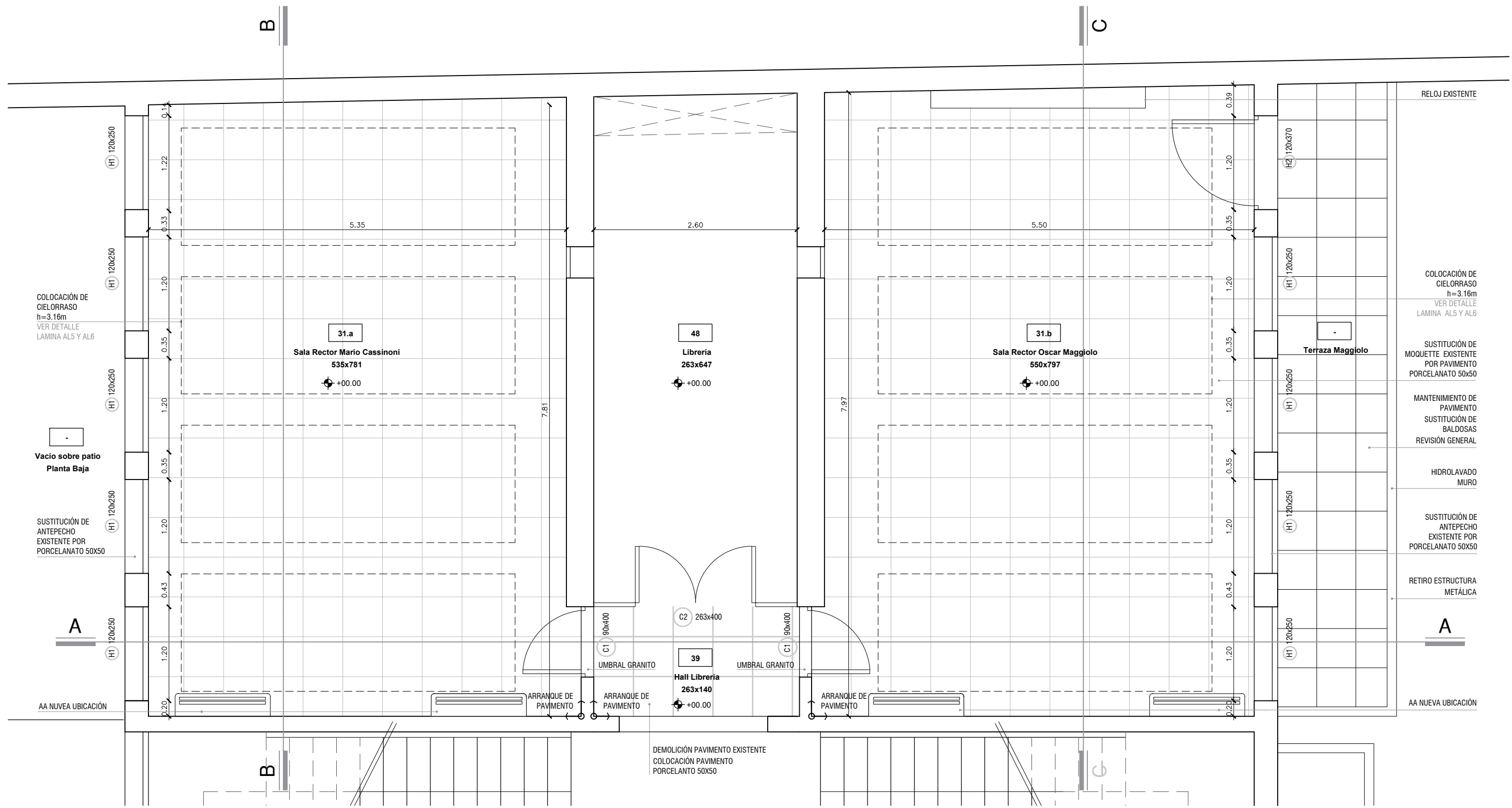
PLANTA SALONES esc. 1:50
