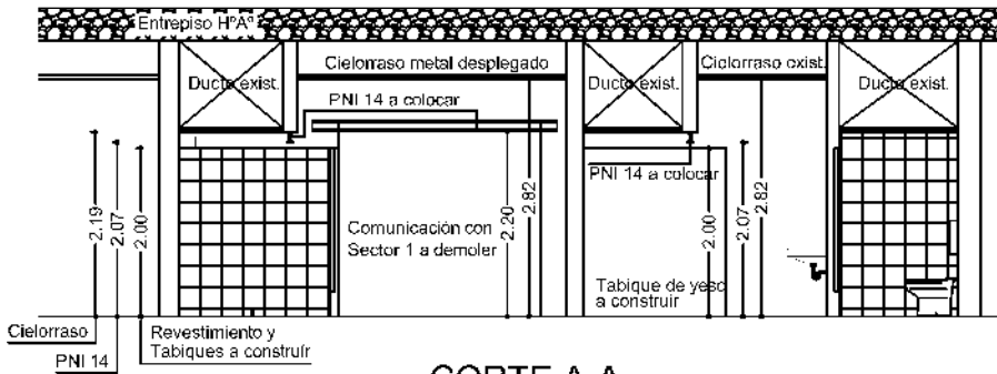
CORTE A-A
