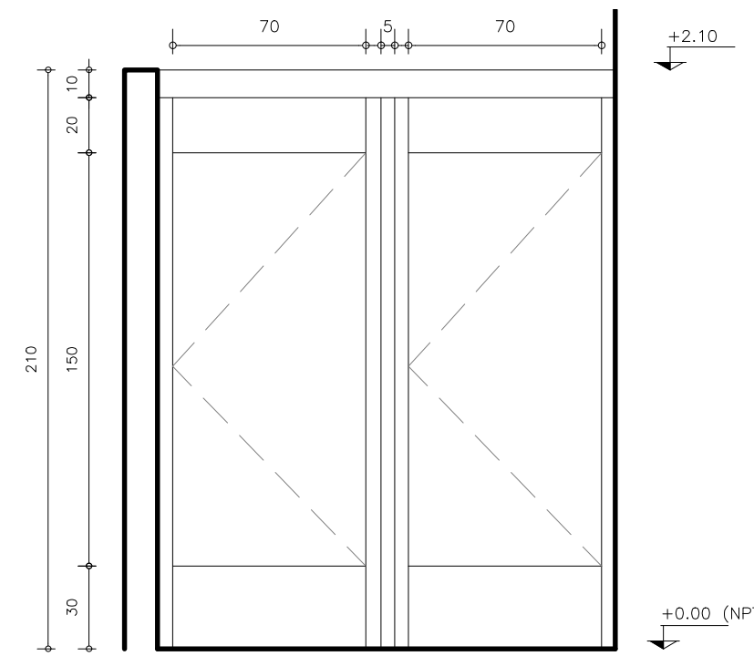
ALZADO esc 1/25
