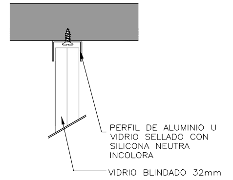
Detalle 1 Escala 1/5
