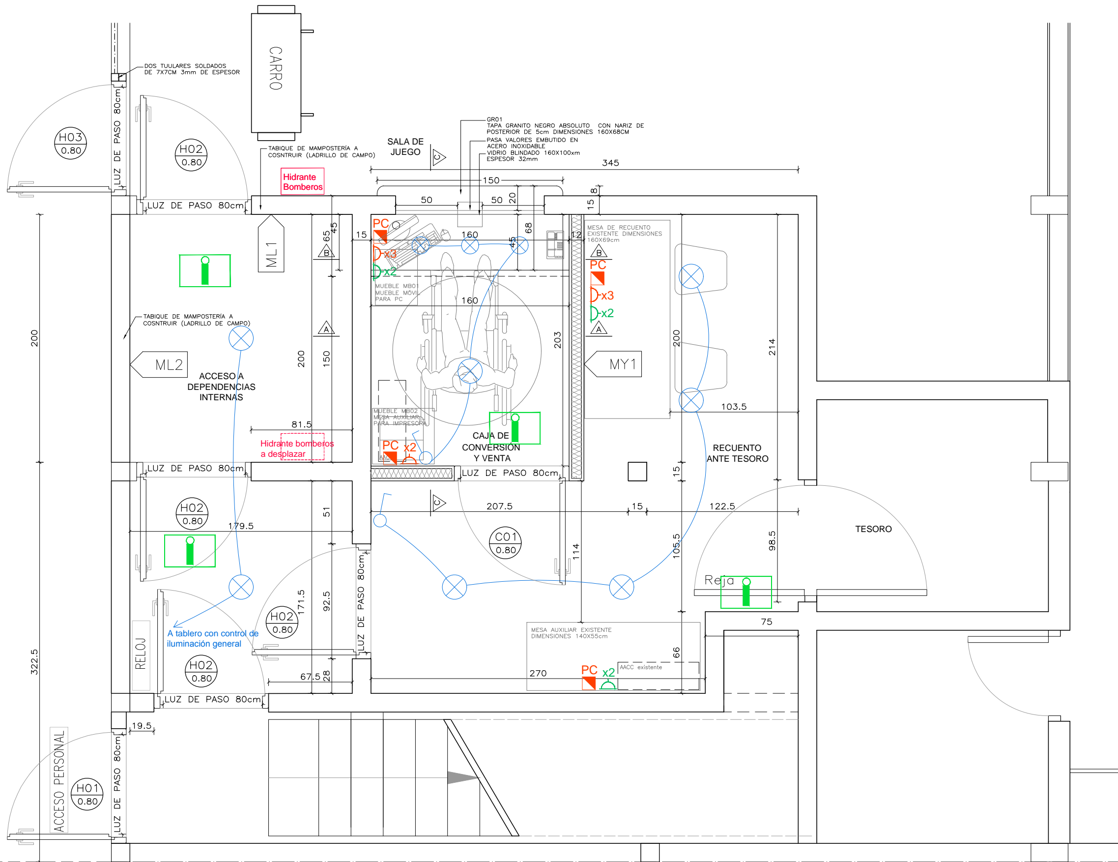
Planta Escala 1/20
