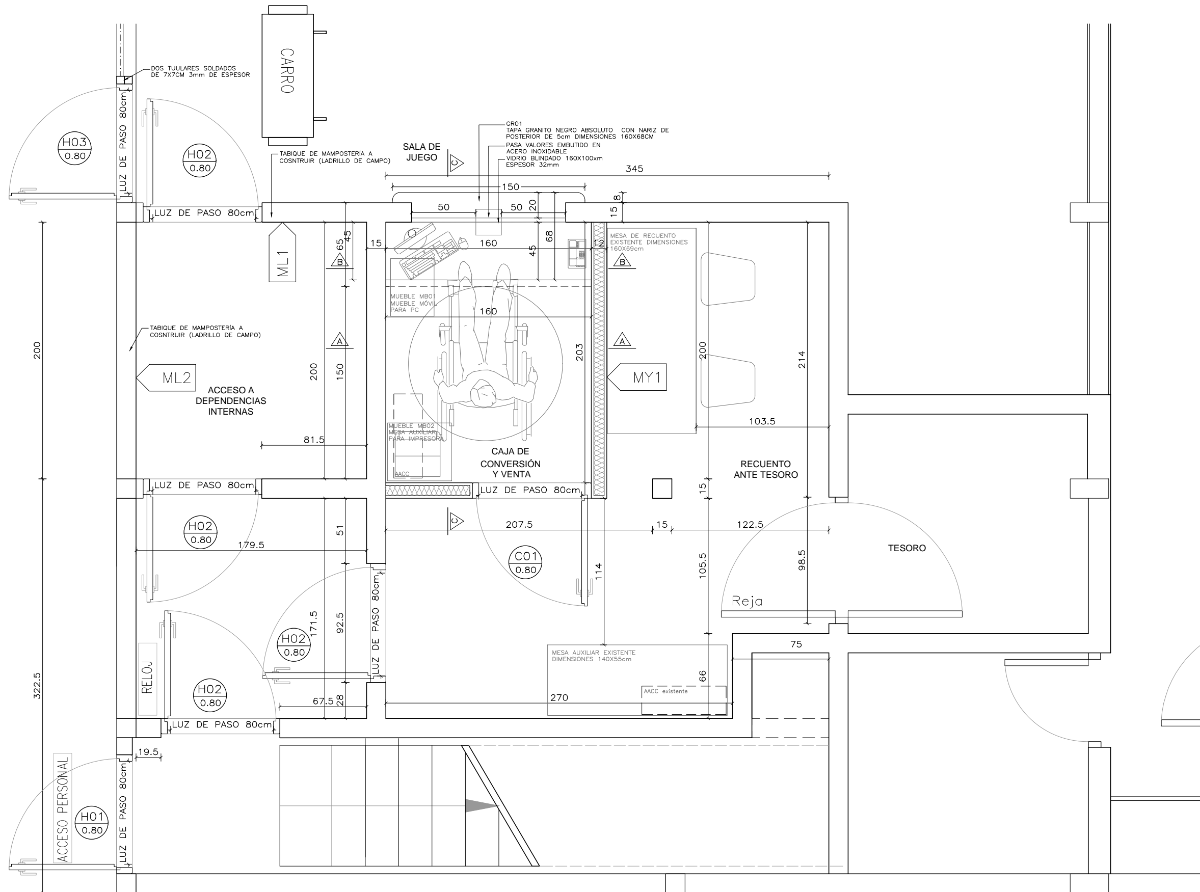
Planta nivel 1 Escala 1/30
