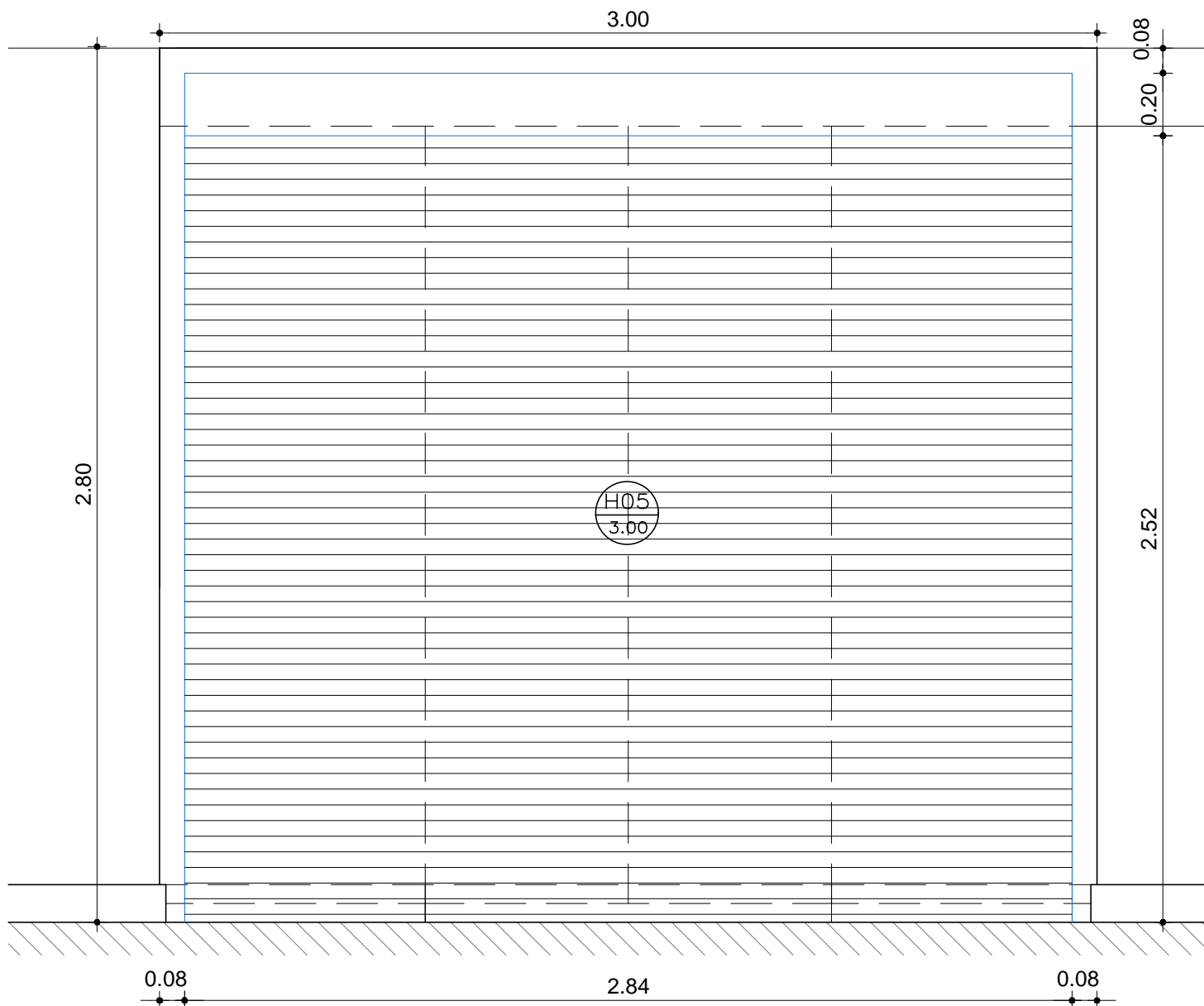
Fachada Escala 1/20
