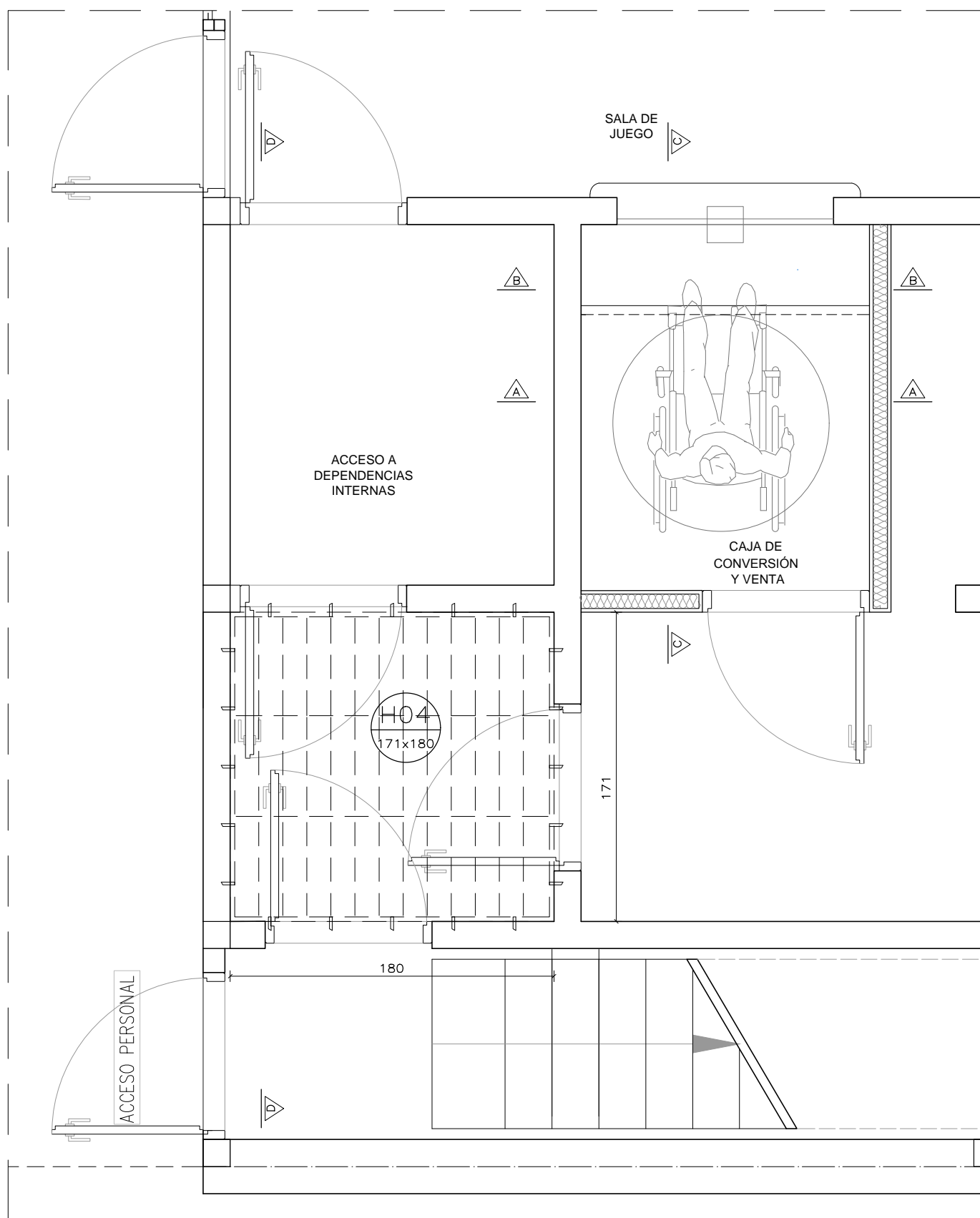
Planta Sector de acceso a nucleo de valores Escala 1/30
