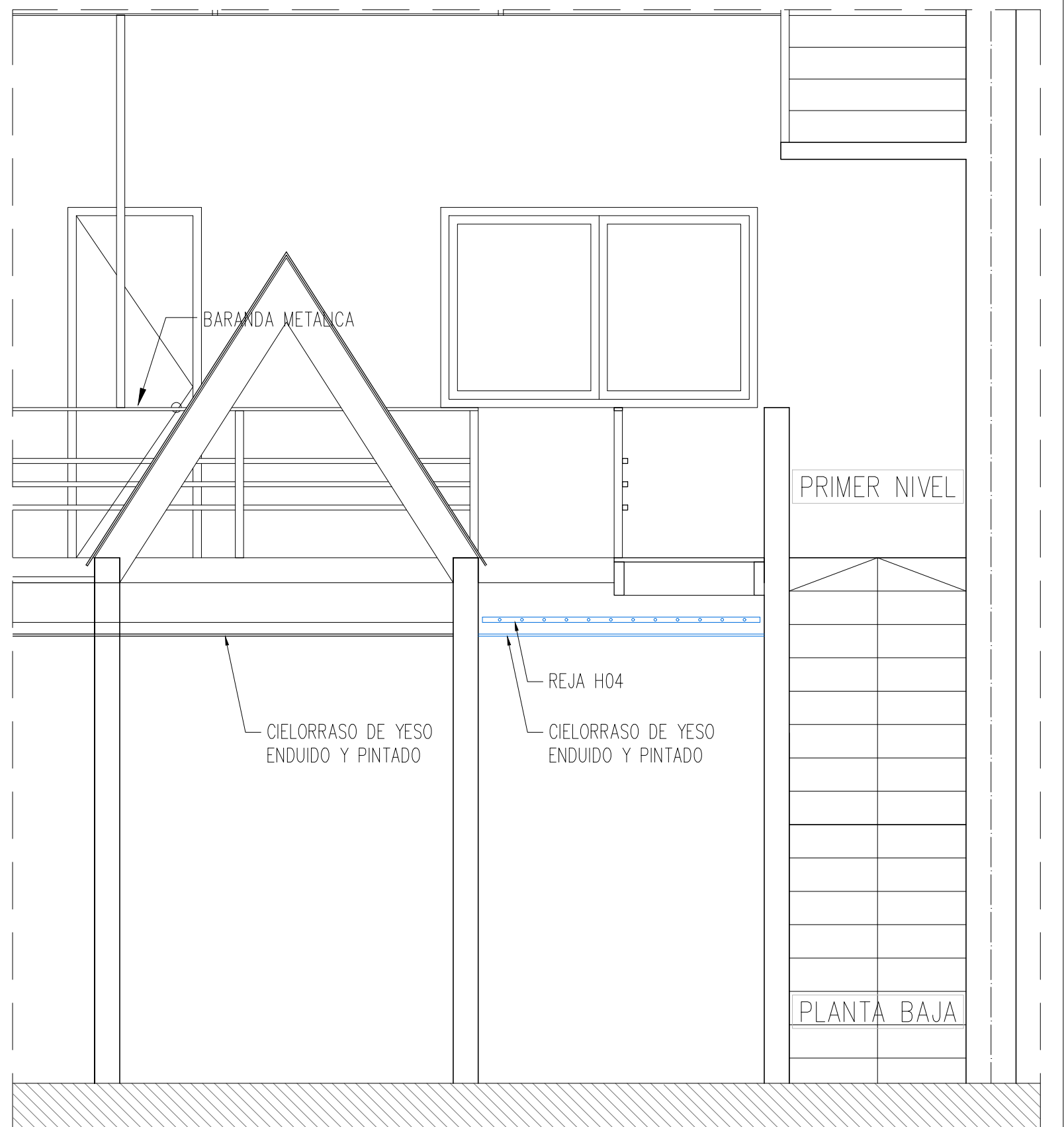
Corte DD Sector de acceso a nucleo de valores Escala 1/30
