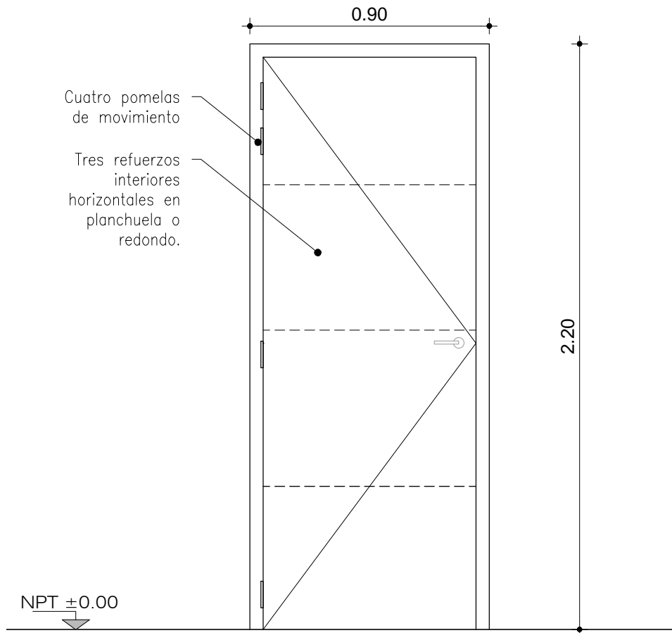
Fachada Escala 1/20
