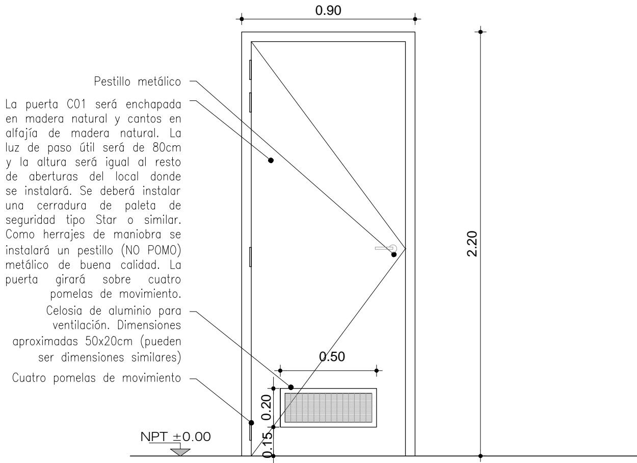
Fachada Escala 1/20
