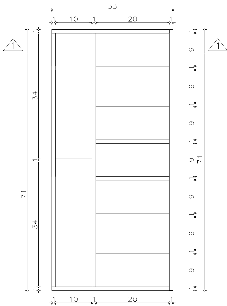
Planta cajón de billetes MB04 Escala 1/5
