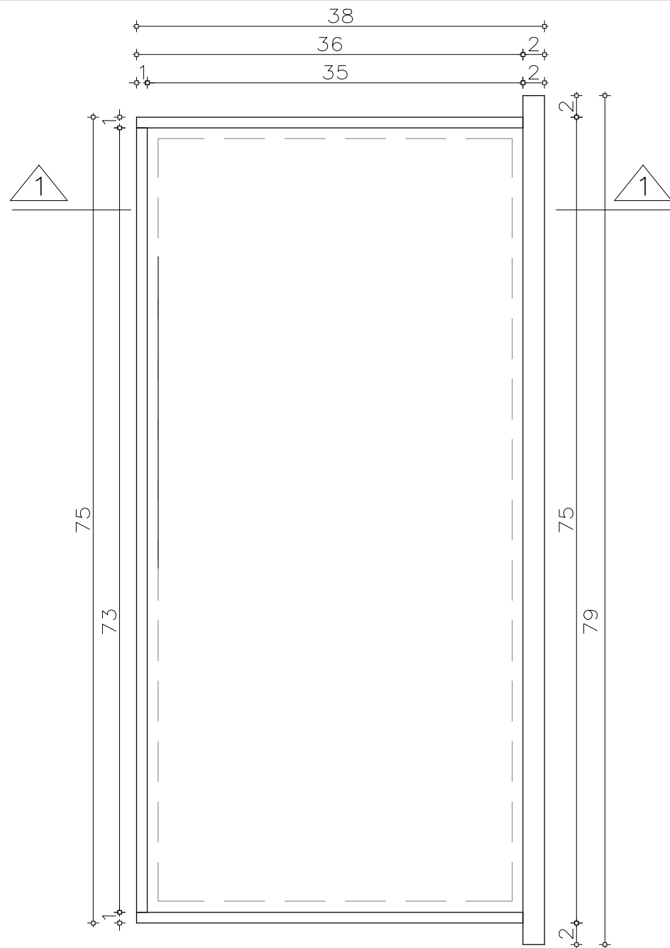
Planta cajón MB03 Escala 1/5
