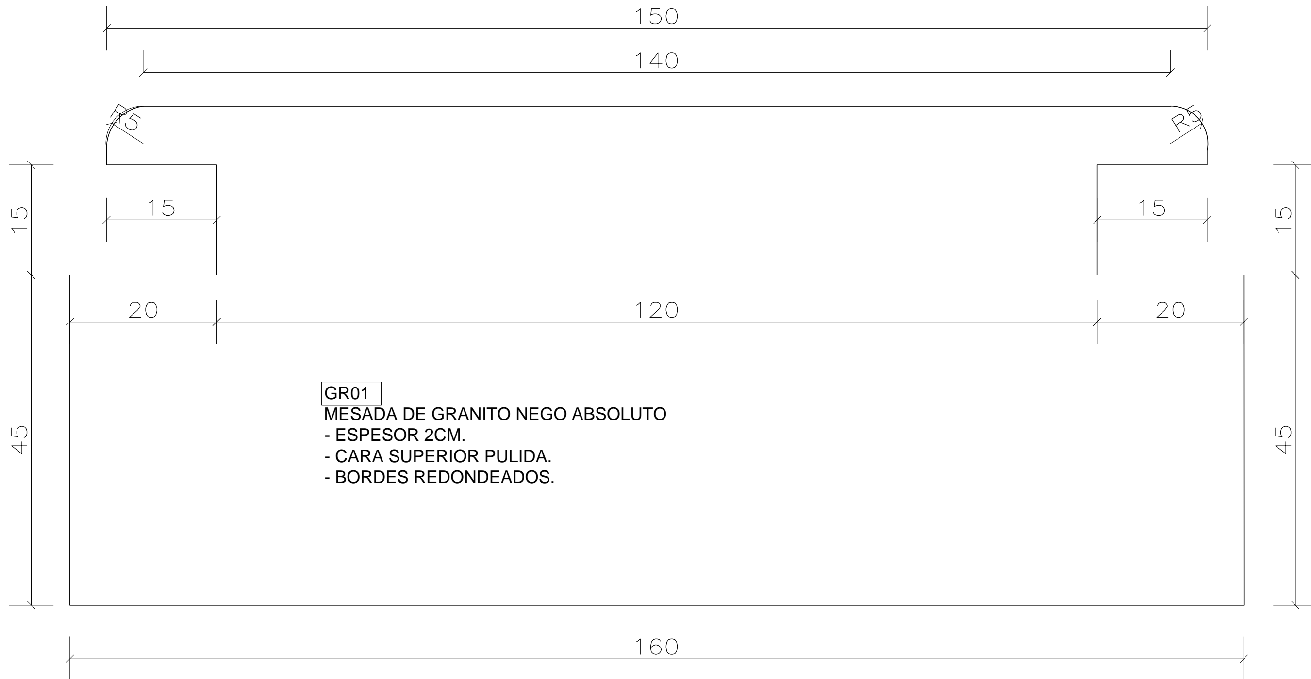
Plano de mesada de atención al público. Escala 1/5 Medidas en cm
