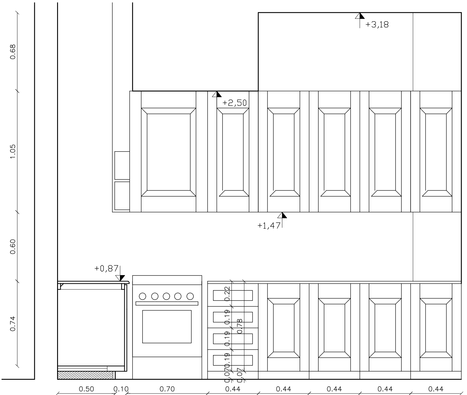
ALZADO NORTE esc : 1/20
