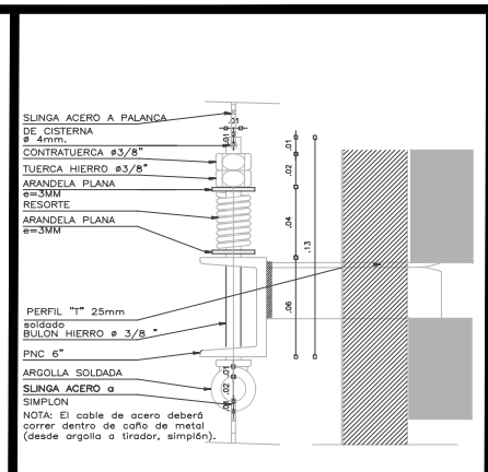
Tirador y conexión de cisterna Esc.: 1:5
