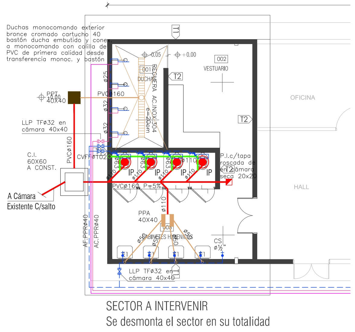
SECTOR A esc. 1./75
