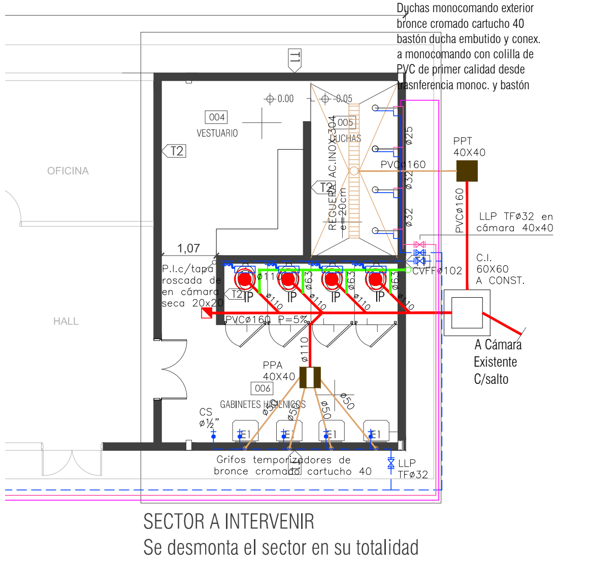
SECTOR B esc. 1./75
