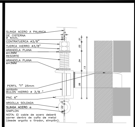
Tirador y conexión de cisterna Esc.: 1:5
