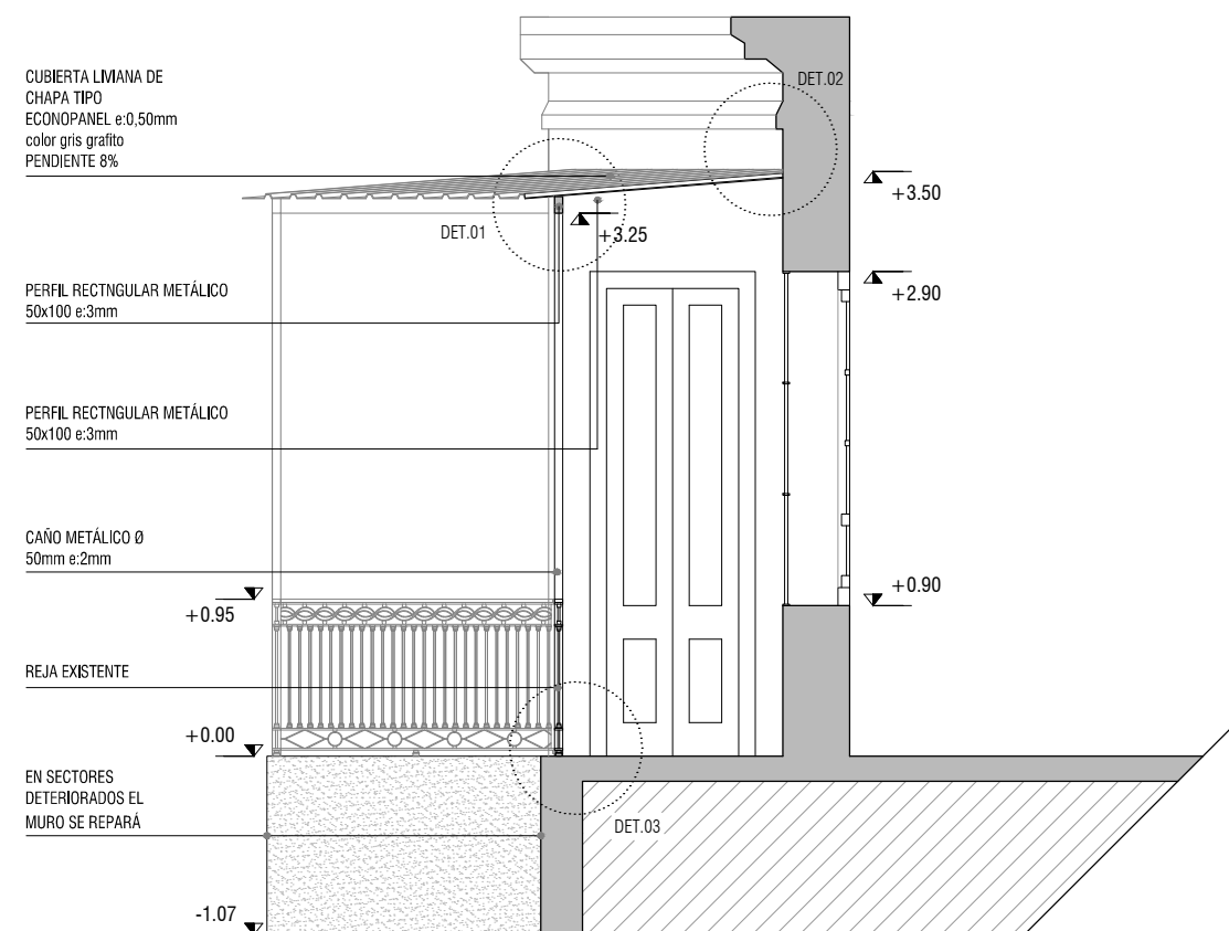
CORTE AA Esc 1/50 PROYECTO
