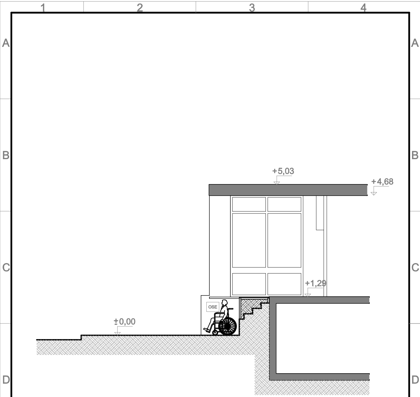
CORTE A-A
