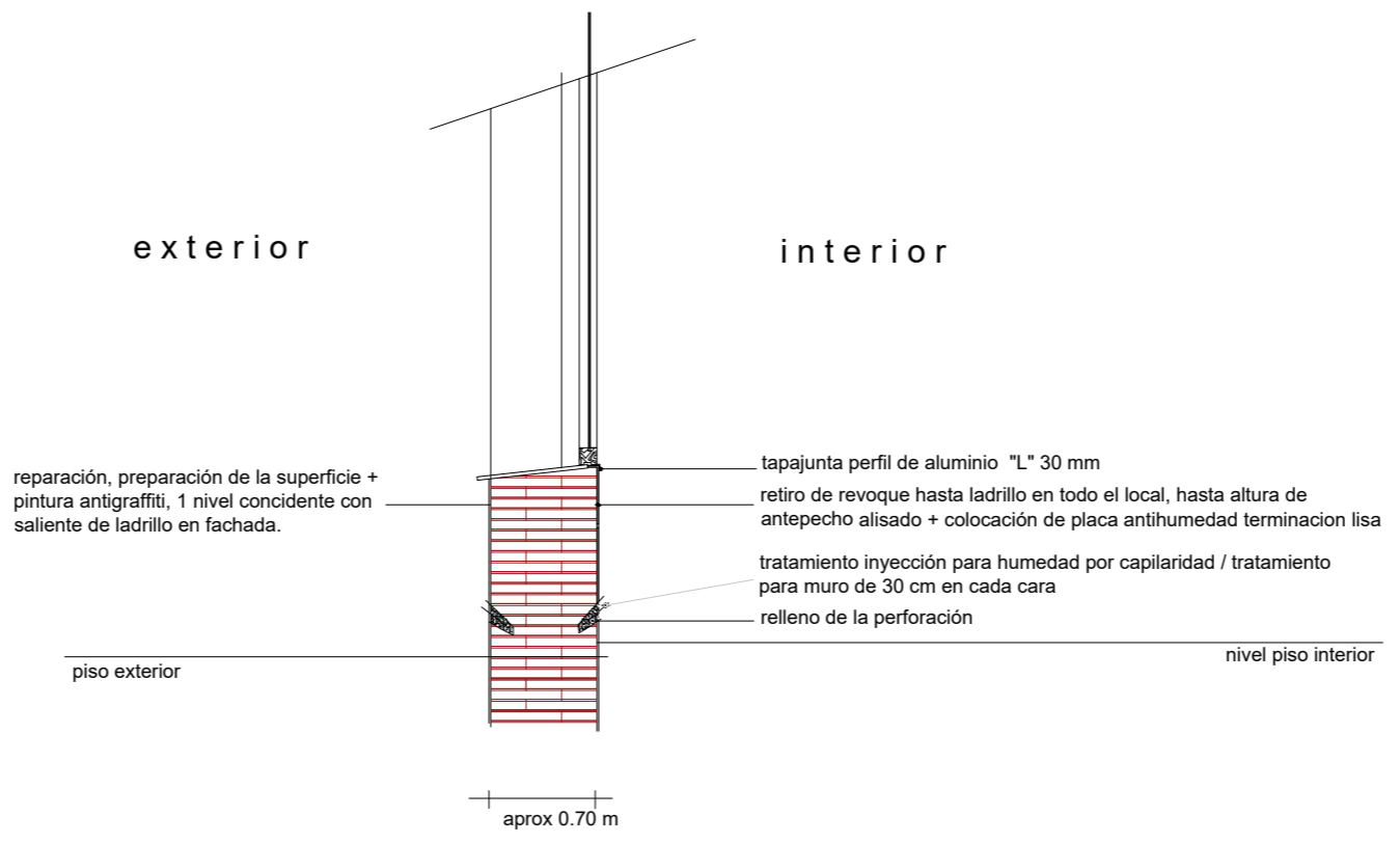
Detalle tratamiento en muro Fachada calle Lauro Müller
