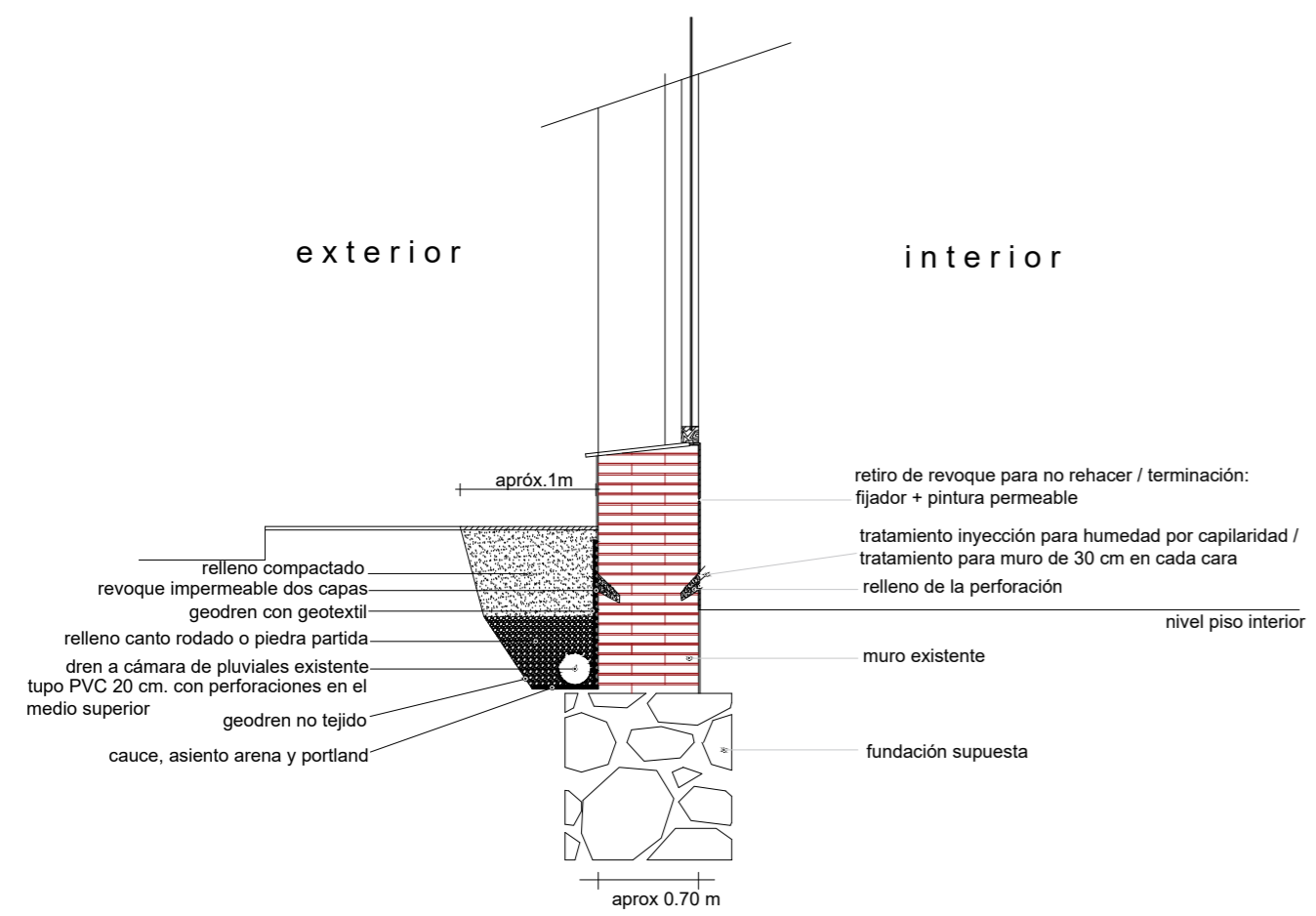
Detalle tratamiento en muro semienterrado Fachada calle Jackson
