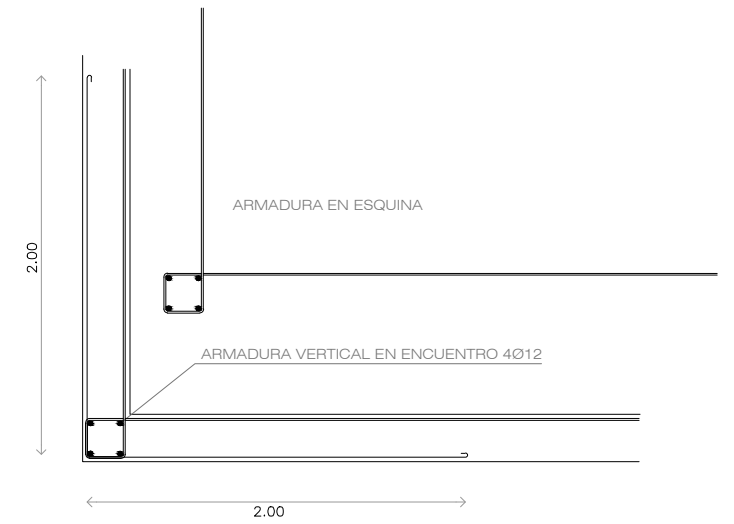
DETALLE 03
