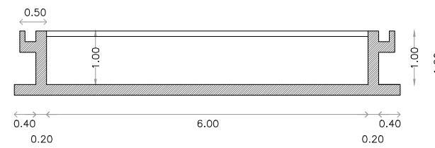
CORTE B-B
